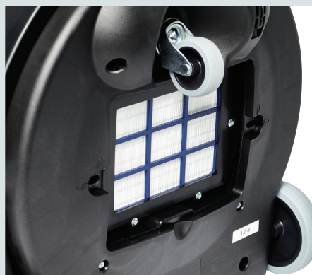
HEPA H13 uitblaasfilter voor een maximaal filtratieniveau om de luchtkwaliteit in de te reinigen ruimte te waarborgen
