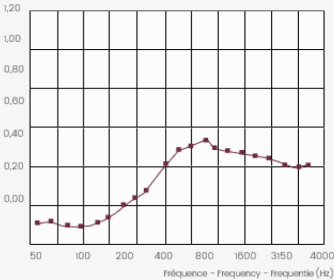
(a) Performance de la matière à absorber les ondes sonores Soundwave absorption effectiveness of a given material Capaciteit van het materiaal om geluidsgolven te absorberen
