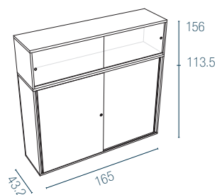
2 melamine schuifdeuren Opzetelement met 2 Altuglas® deuren
